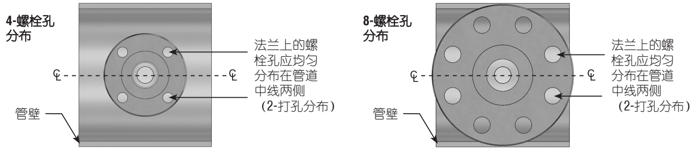
图 4. 法兰方向
